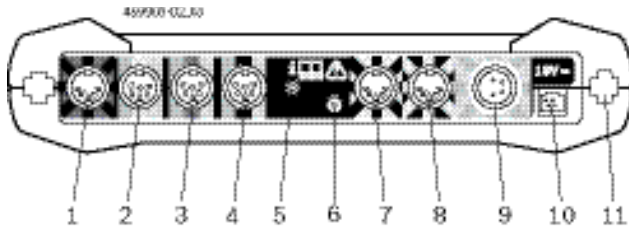
Fig. 2: FSA 500 панель подключений (вид снизу)
