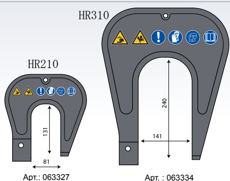
Набор плеч HR210 + HR310 Арт. : 064089
